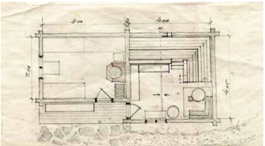
Metsästysmajan ja saunan suunnittelijan, kajaanilaisen arkkitehdin, luutnantti Eino Pitkäsen luonnos saunasta. Kuvat SMMM arkisto.
